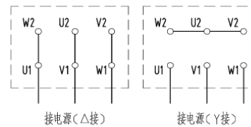
电动机主电源接线图
